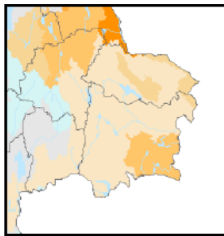
Figur 3: Antal dagar med lågflöde (torrare klimat) beräknat för år 2098.
